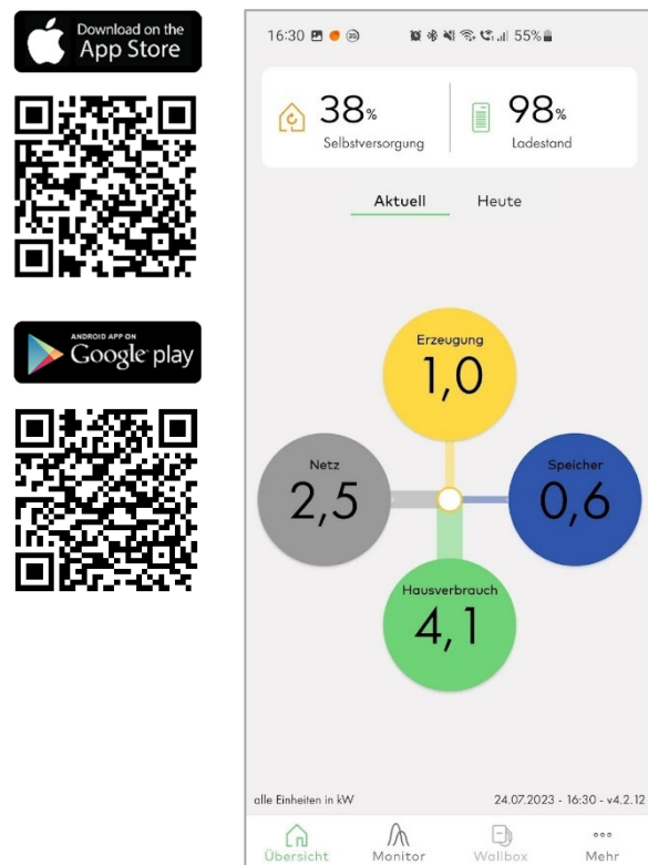
5: Beispielansicht APP
